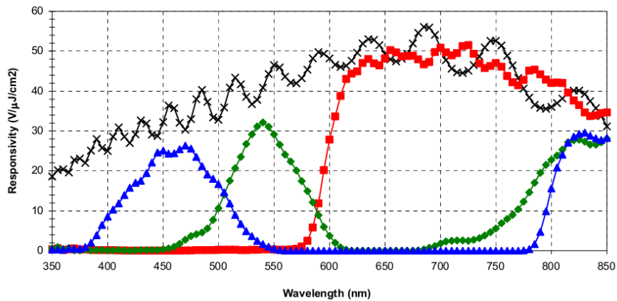
OK_LC2060 光谱曲线
